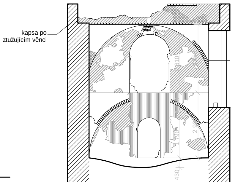
SEVEROVÝCHODNÍ ZEĎ M 1:100
