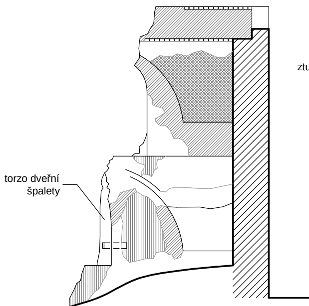
SEVEROZÁPADNÍ ZEĎ M 1:100
