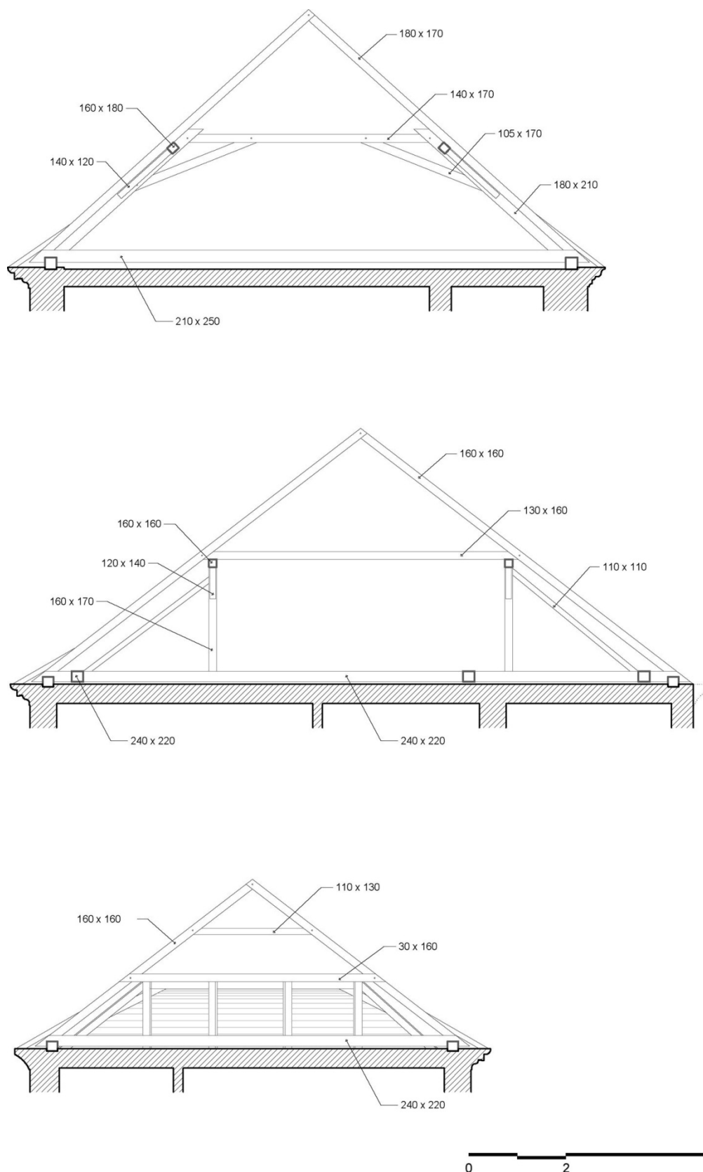
▲ Obr. 27: Schéma plných vazeb krovu. Nahoře tzv. Rankův krov z poloviny 19. století nad jižní částí východního křídla, uprostřed hambálkový krov z 1. poloviny 19. století nad severním a částí východního křídla, dole hambálkový krov s nosnou konstrukcí falešné klenby nad západní částí severního křídla.
