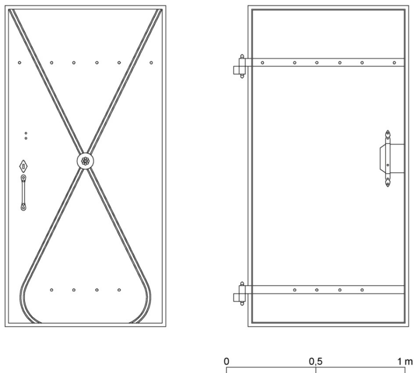
▲ Obr. 29: Pohled na líc a rub železných dveří z počátku 20. století ve vstupu do krovu.
