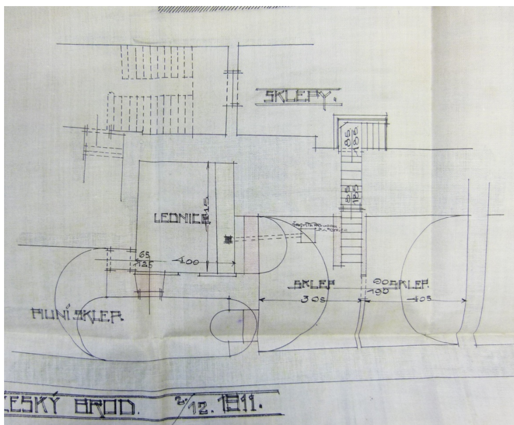
▲ Obr. 21: Detail půdorysu sklepů z plánu stavebních úprav střední části domu z roku 1911.
