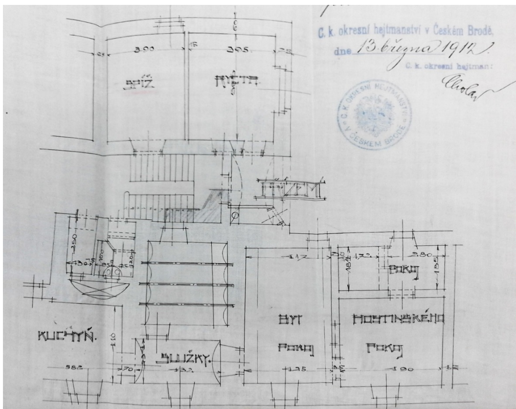
▲ Obr. 20: Detail půdorysu přízemí z plánu stavebních úprav střední části domu z roku 1911.
