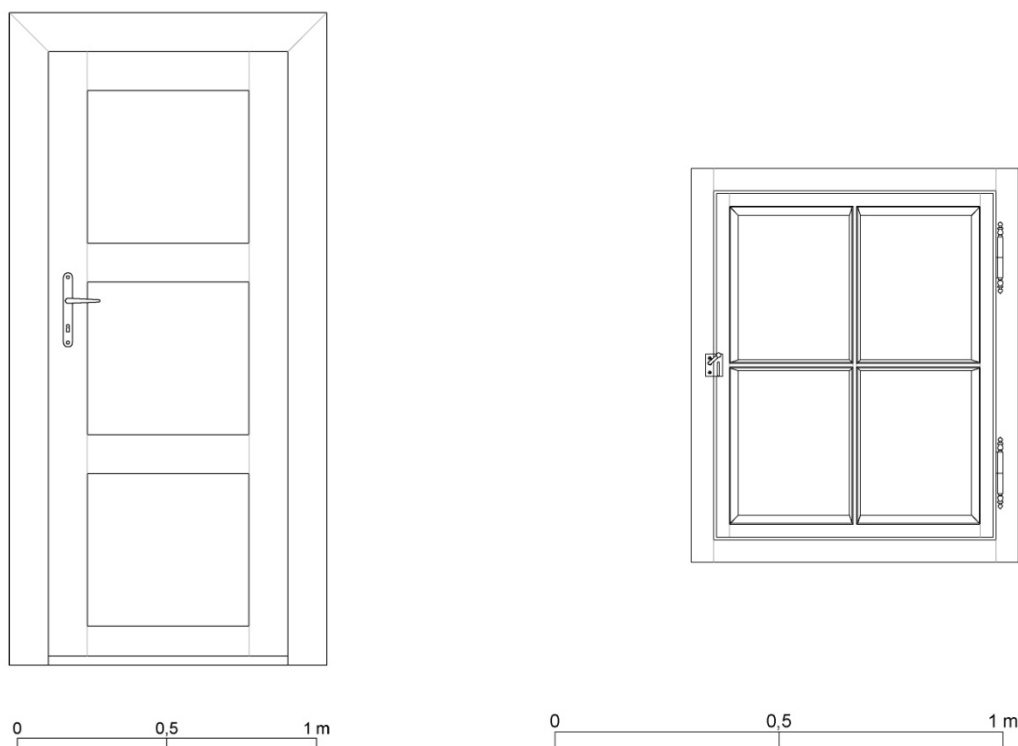
▲ Obr. 30: Vlevo lícová strana dveří ze 40. let 20. století v místnosti P08. Vpravo okno světlíku v prostoru krovu z počátku 20. století.
