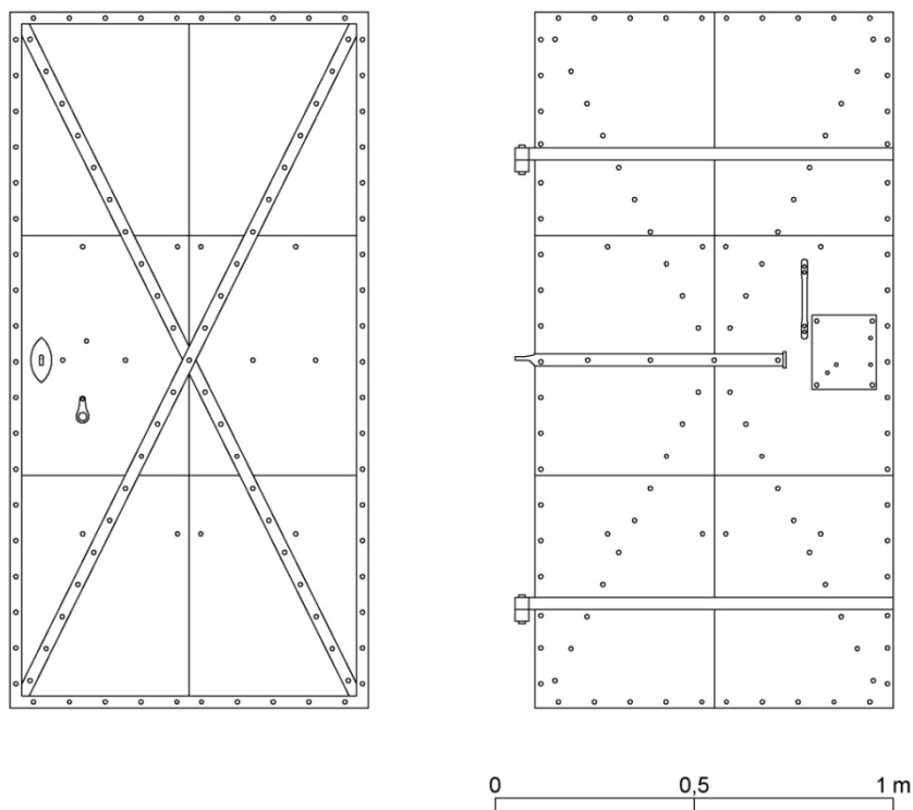
▲ Obr. 28: Pohled na líc a rub železných dveří z poloviny 19. století ve štítové zdi krovu.
