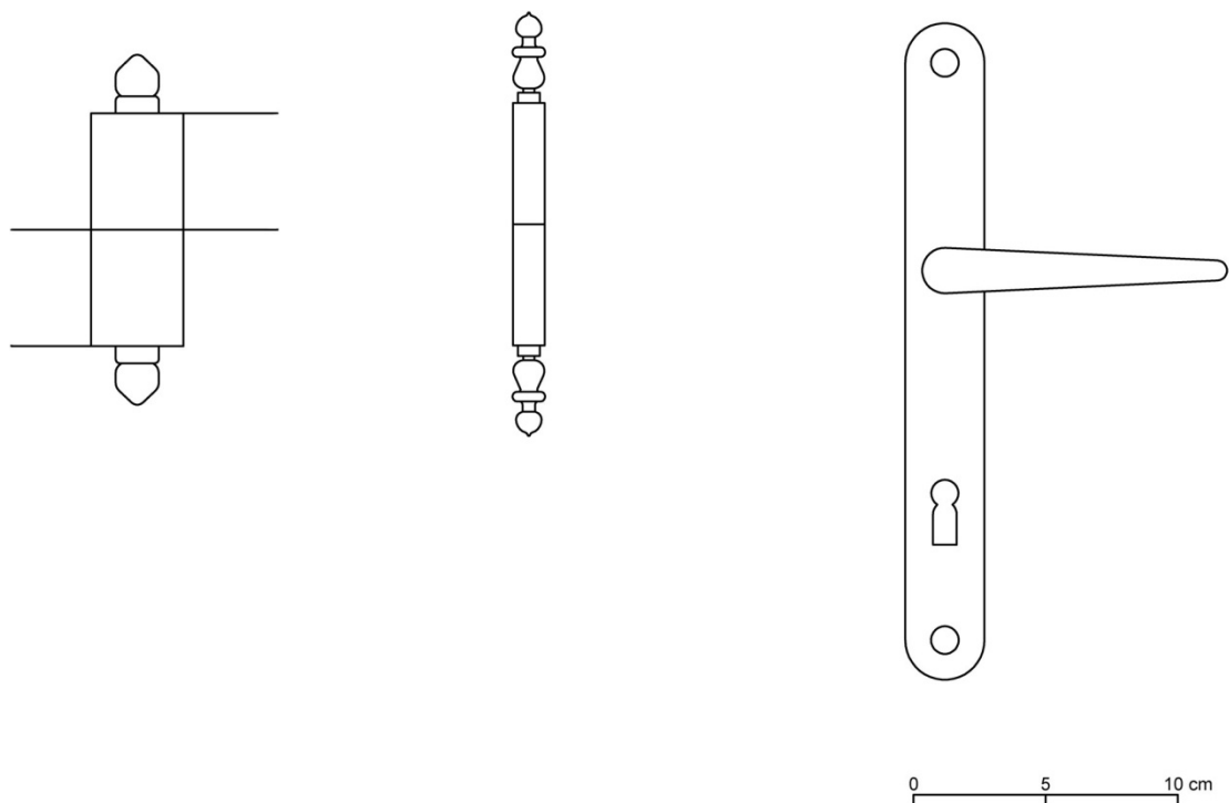
▲ Obr. 31: Detaily kování. Vlevo kování s žaludovými konci železných dveří do krovu datovatelné do počátku 20. století. Uprostřed zapuštěný závěs okna šachty v prostoru krovu s bohatými „barokními“ profily konců z počátku 20. století. Vpravo jednoduše tvarovaná dvevní klika z bílé slitiny ze 40. let 20. století na dveřích v místnosti P08.
