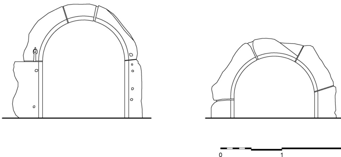
▲ Obr. 25: Vlevo portál s polodrážkou ve sklepe S06 pravděpodobně z 16. století, vpravo gotický portál s okosením ve sklepe S09 z počátku 15. století.
