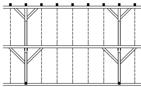
▲ Schéma vazby mladšího krovu severního křídla datovatelného do 20. let 20. století.
