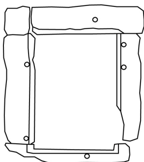
▲ Detaily okenních ostění budovy na západním průčelí severního křídla. Vlevo renesanční kamenné ostění z poloviny 16. století, vpravo vrcholně barokní ostění z 1. poloviny 18. století.
