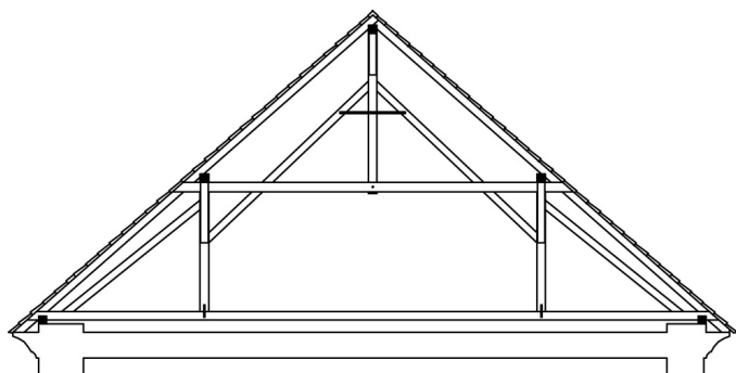
▲ Schéma vazby mladšího krovu severního křídla datovatelného do 20. let 20. století.
